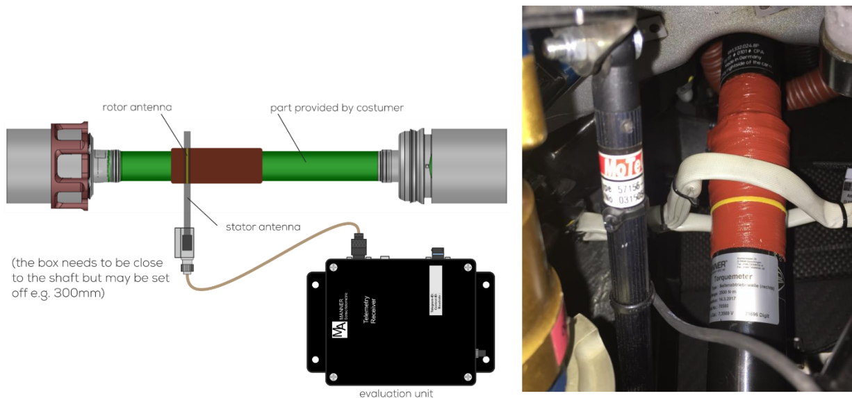
Abbildung 2 Systemüberblick
